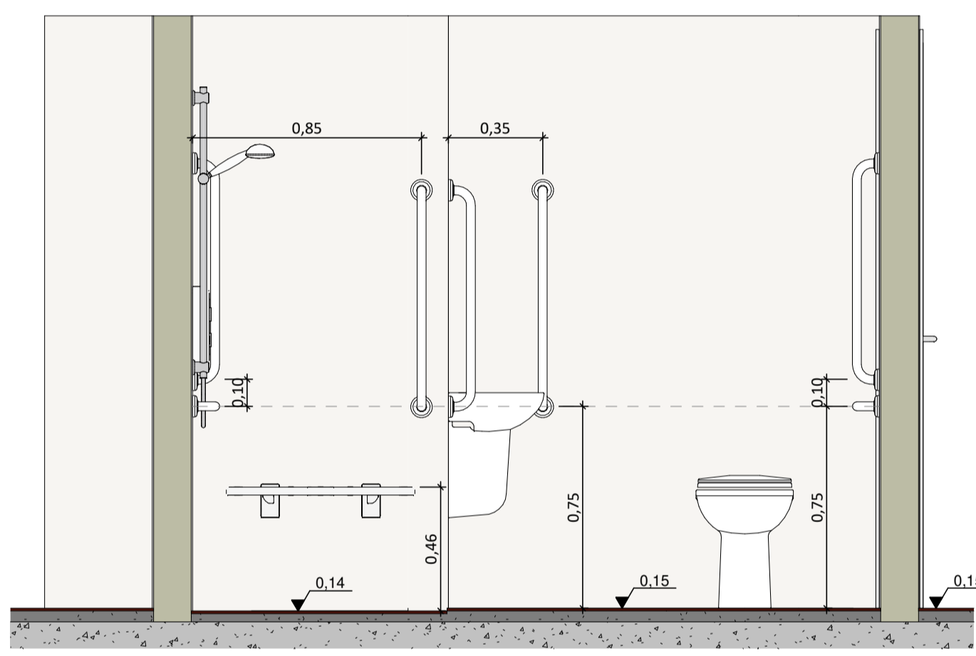
C1 VESTIBULÁRIOS - CORTE - C1 ESC 1:20
