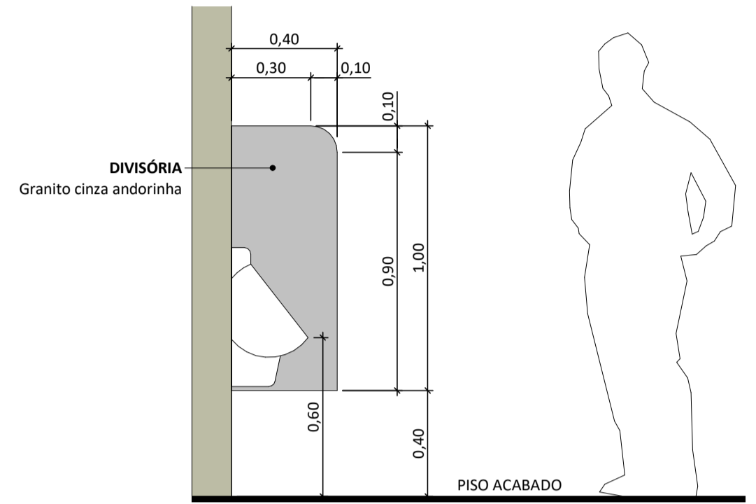
4 VESTIBULÁRIOS - DETALHE - MICTÓRIOS ESC 1:20
