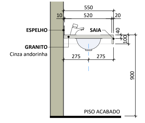
6 VESTIBULÁRIOS - DETALHE - BANCADA ESC 1:20 *dimensões em milímetros
