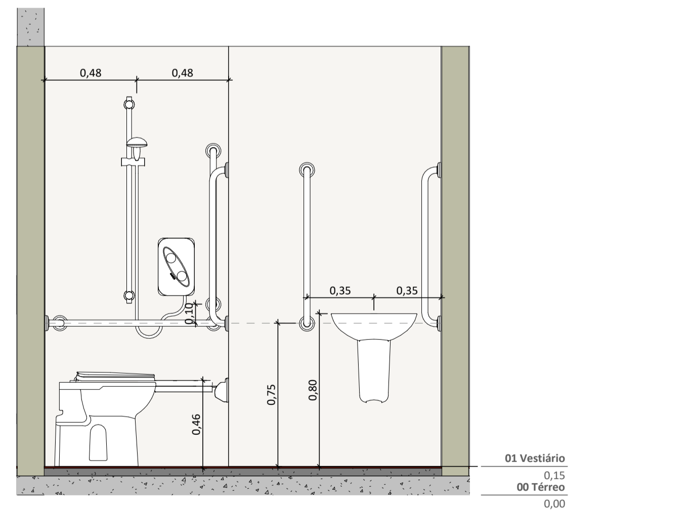
C2 VESTIBULÁRIOS - CORTE - C2 ESC 1:20
