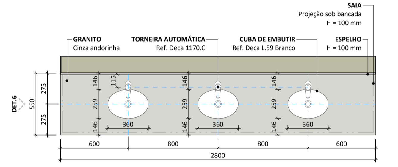
5 VESTIBULÁRIOS - DETALHE - BANCADA ESC 1:20 *dimensões em milímetros
