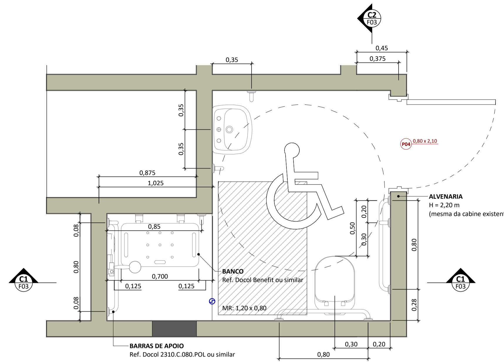
2 VESTIBULÁRIOS - BANHEIROS PNE ESC 1:20
