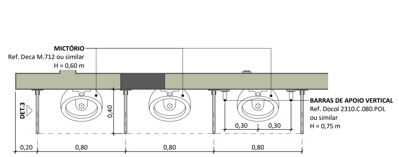
3 VESTIBULÁRIOS - DETALHE - MICTÓRIOS ESC 1:20
